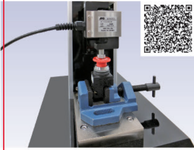
包装容器の圧縮強度試験
