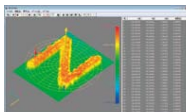
面の幾何偏差作図
