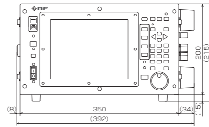
正面図(フロントカバーなし)
