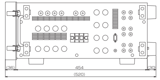
右側面図 (端子保護カバーなし)
