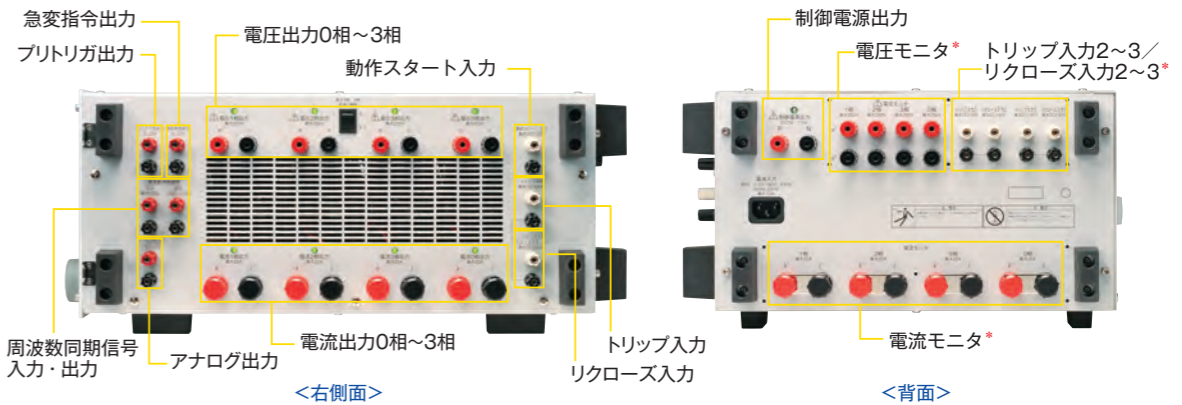
<右側面>
