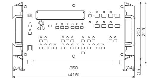
正面図 (フロントカバーなし)
