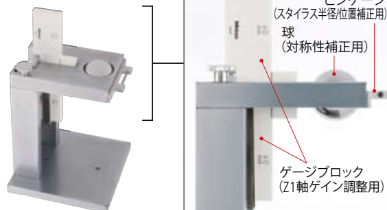
ピンゲージ (スタイラス半径位置補正用)
